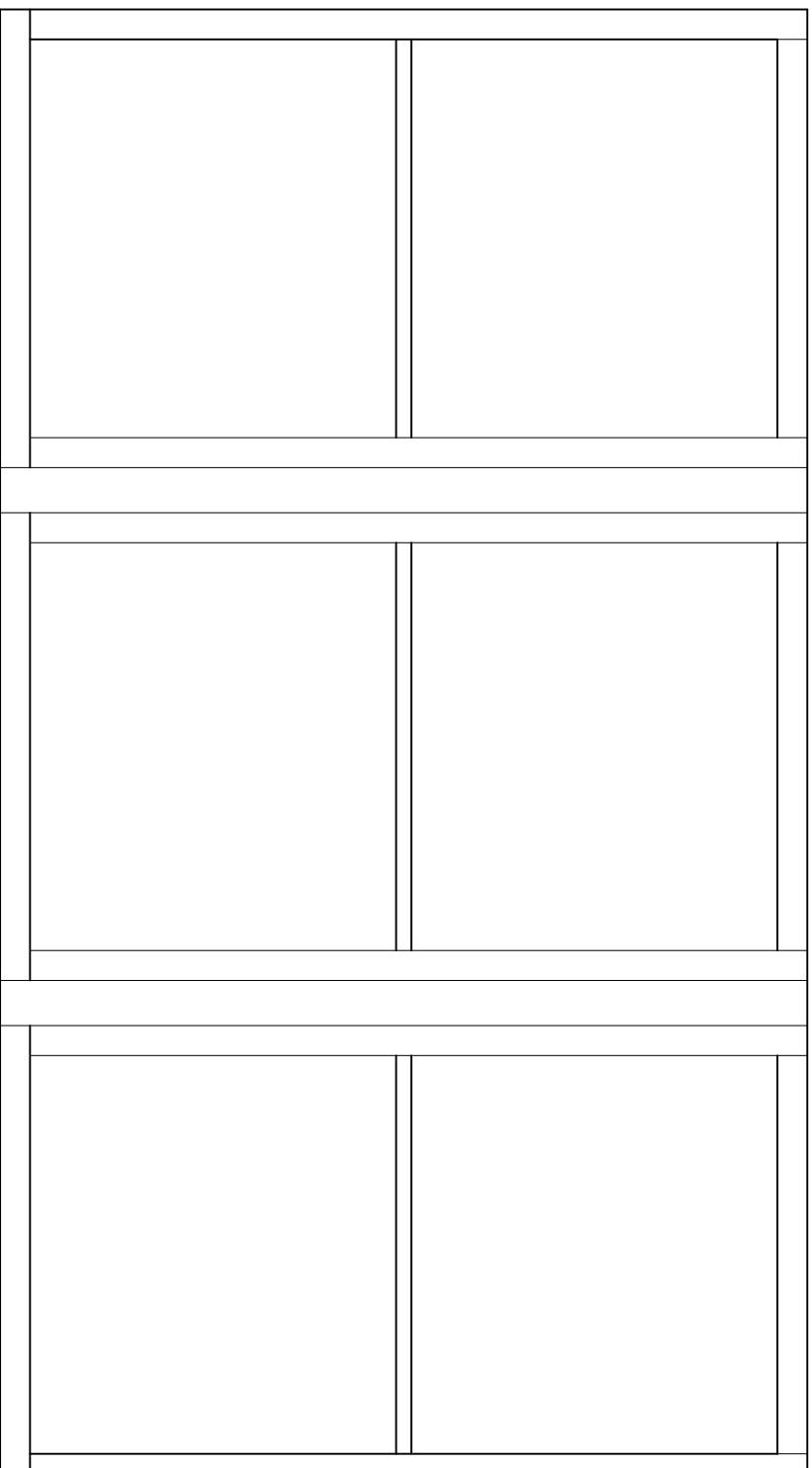
Widok nowo projektowanego okna E od frontu, skala 1:10
